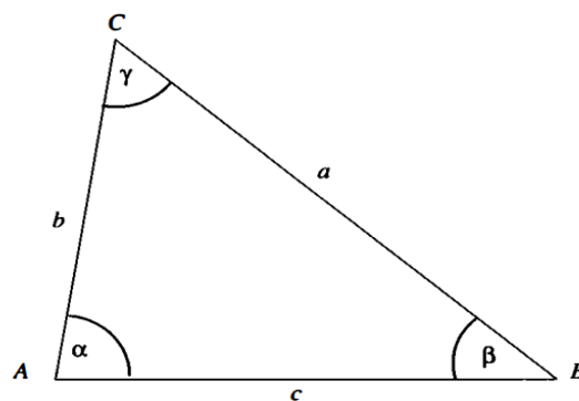
Slika 1: Trokut ABC
