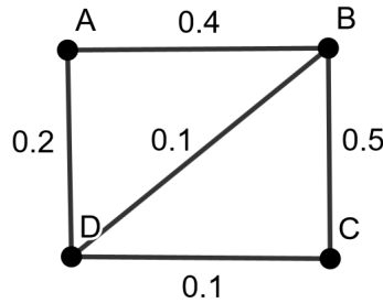
Slika 1: Fuzzy graf G
